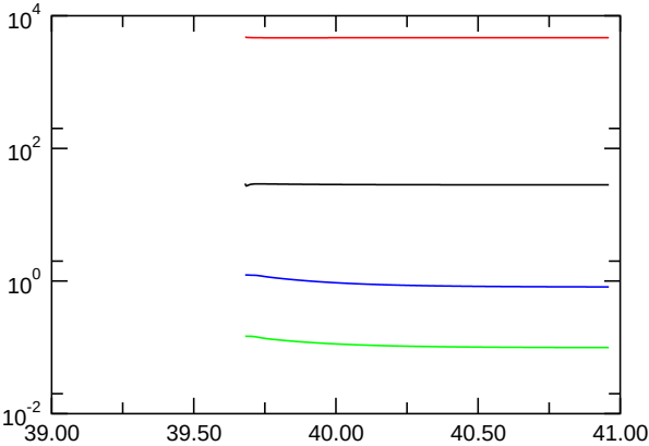
E_{kin,symm.}
