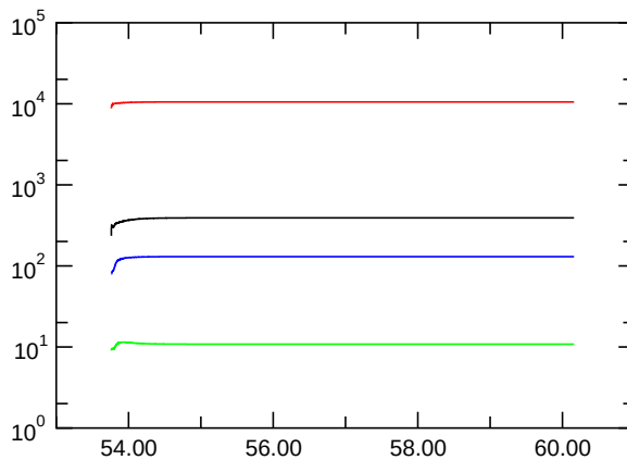
E_{\text{kin,symm.}}
