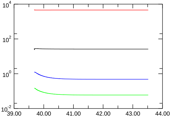
E_{\text{kin,symm.}}
