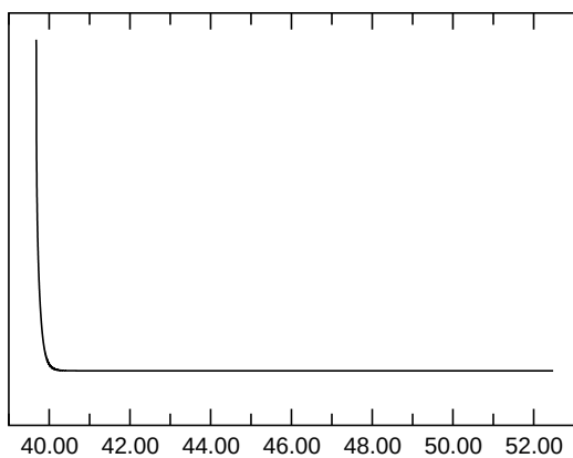
E_{\text{kin,asymm.}}
