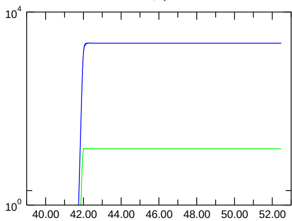
E_{\text{kin,asymm.}}
