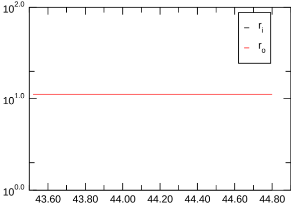
Nusselt Number
