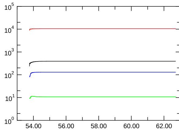
Nusselt Number
