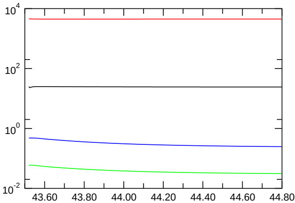
E_{kin,symm.}
