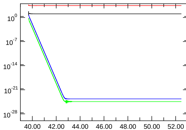
Nusselt Number
