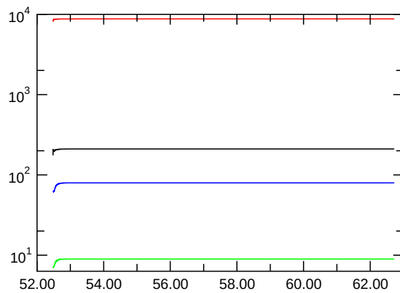
Nusselt Number
