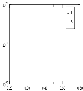
Nusselt Number
