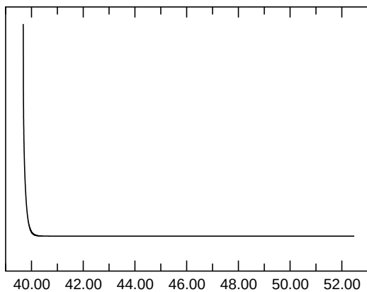
E_{\text{kin,asymm.}}
