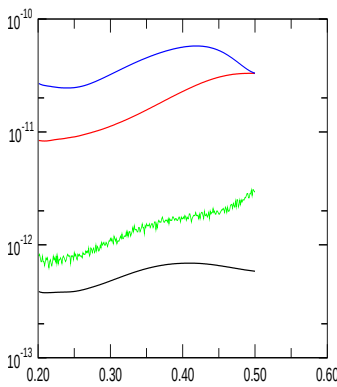
E_{magn,quadr.}
