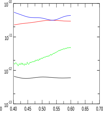
E_{\text{magn,quadr.}}
