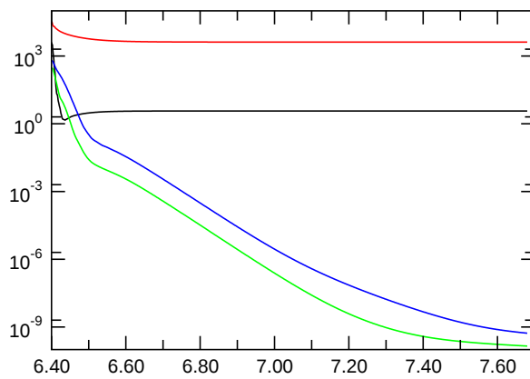
Nusselt Number
