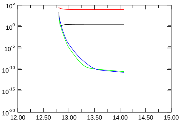
E_{kin,symm.}
