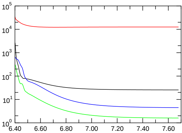
E_{\text{kin,symm.}}
