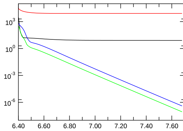
Nusselt Number
