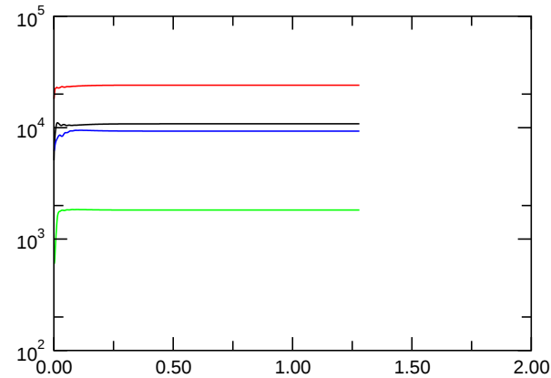
E_{kin,symm.}
