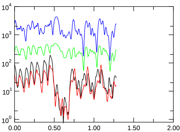
E_{\text{kin,asymm.}}
