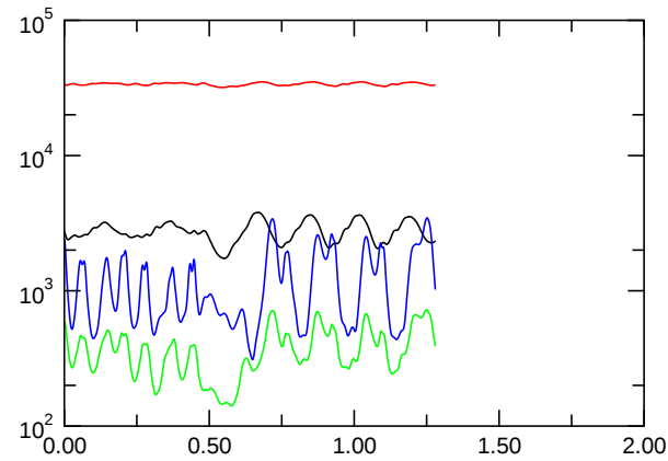
E_{\text{kin,symm.}}
