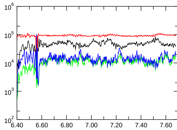
Nusselt Number
