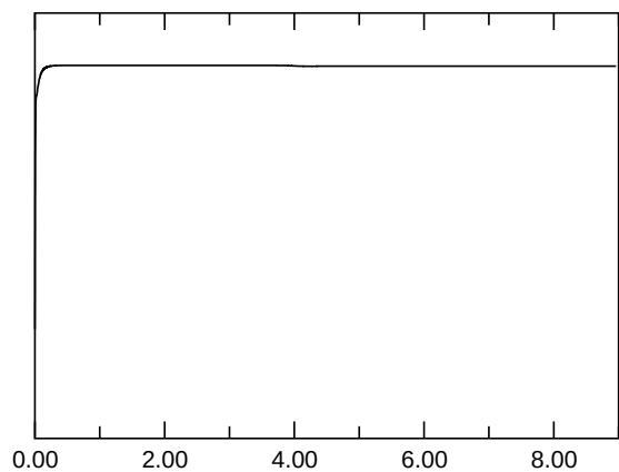
E_{\text{kin,asymm.}}
