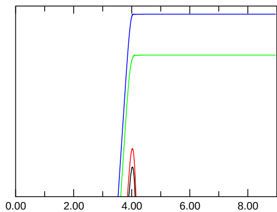
E_{\text{kin,asymm.}}
