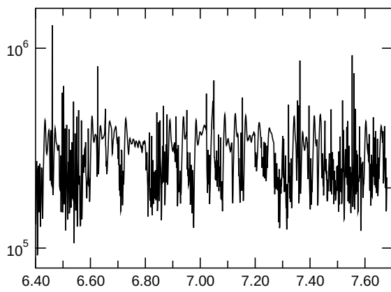
E_{\text{kin,asymm.}}
