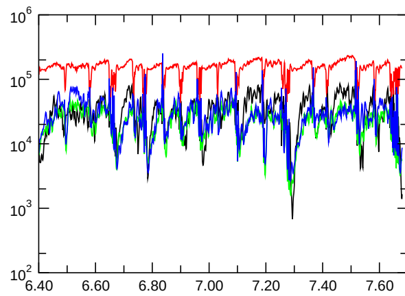
Nusselt Number
