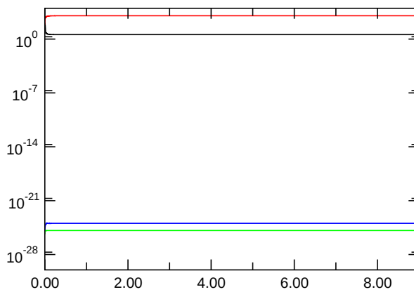
Nusselt Number
