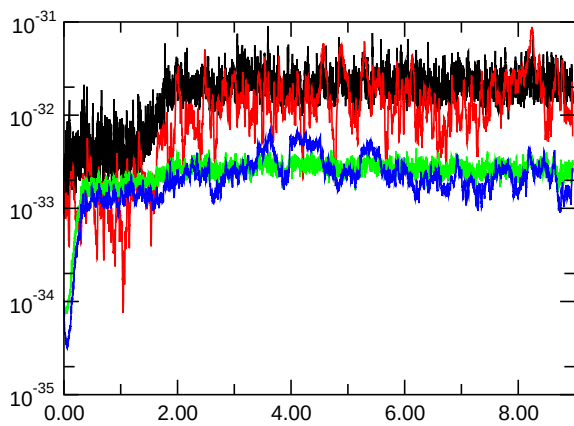
E_{\text{kin,asymm.}}
