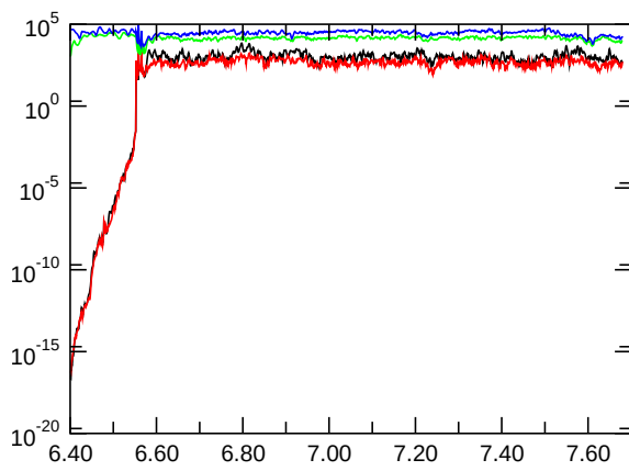
E_{\text{kin,asymm.}}
