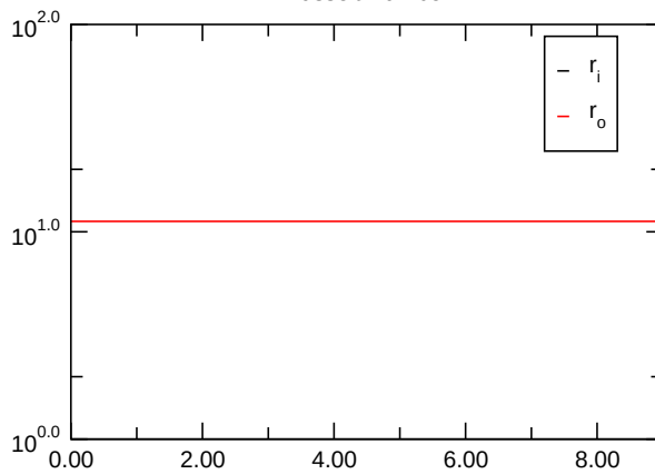
Nusselt Number
