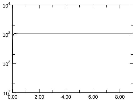
E_{\text{kin,asymm.}}
