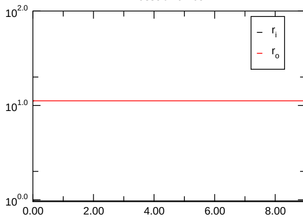
Nusselt Number
