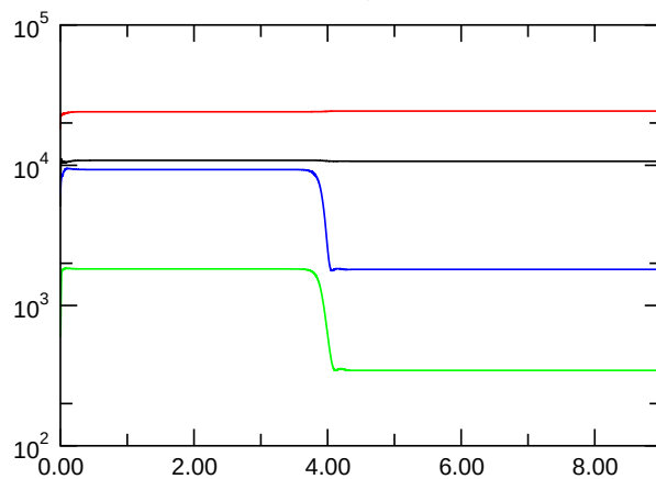
E_{\text{kin,symm.}}
