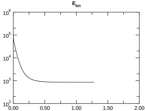
E_{\text{kin,asymm.}}
