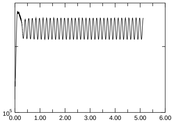
E_{\text{kin,asymm.}}
