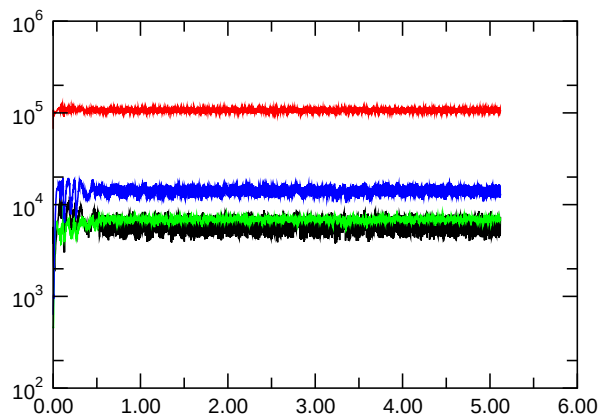
E_{\text{kin,symm.}}
