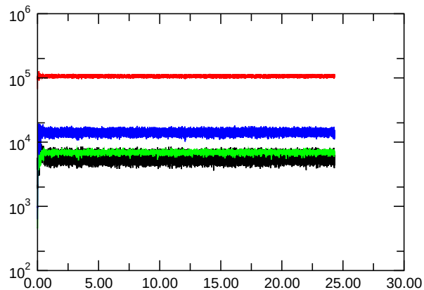
E_{\text{kin,symm.}}
