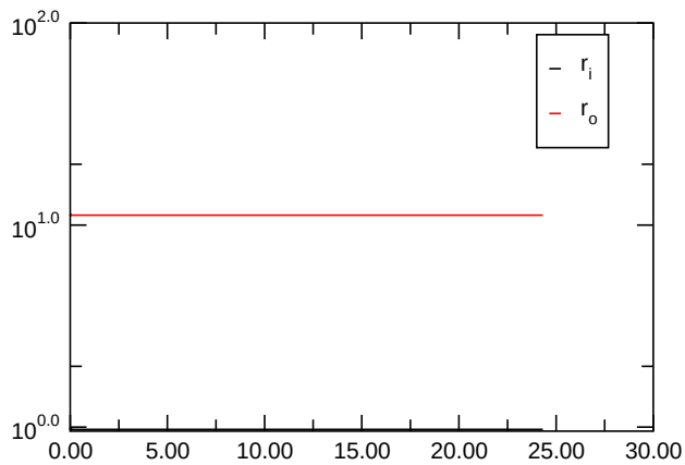
Nusselt Number
