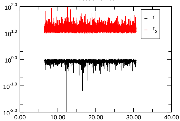
Nusselt Number
