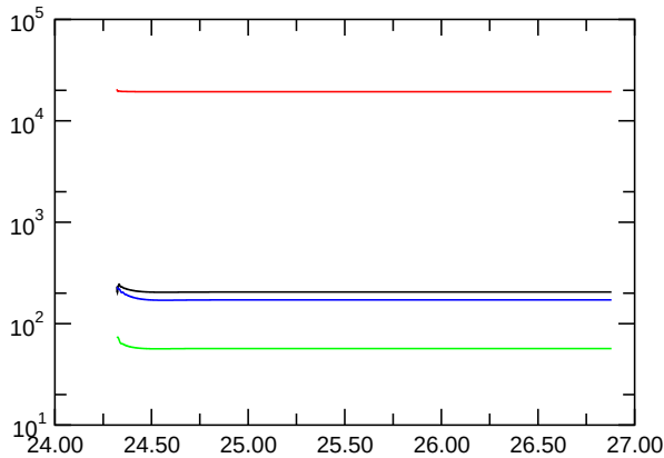
E_{\text{kin,symm.}}
