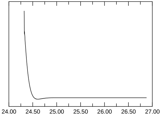
E_{\text{kin,asymm.}}
