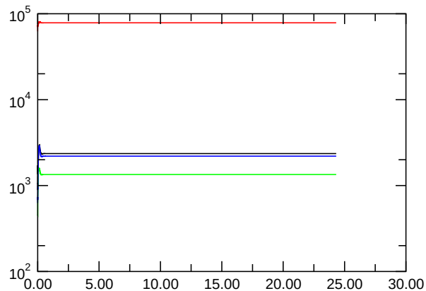
E_{kin,symm.}
