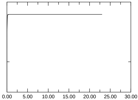
E_{\text{kin,asymm.}}
