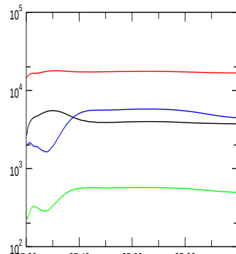
E_{kin,symm.}
