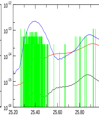
E_{magn,quadr.}
