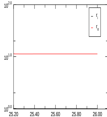
Nusselt Number
