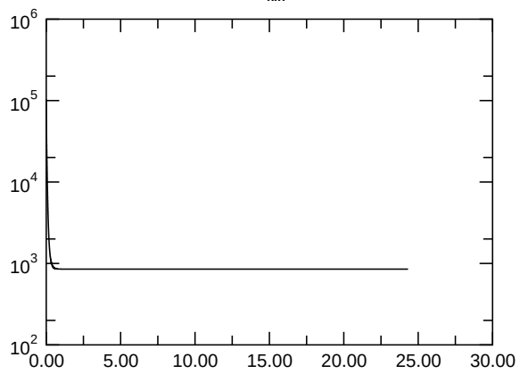
E_{\text{kin, asymm.}}
