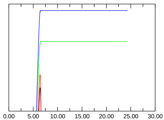
E_{\text{kin, asymm.}}
