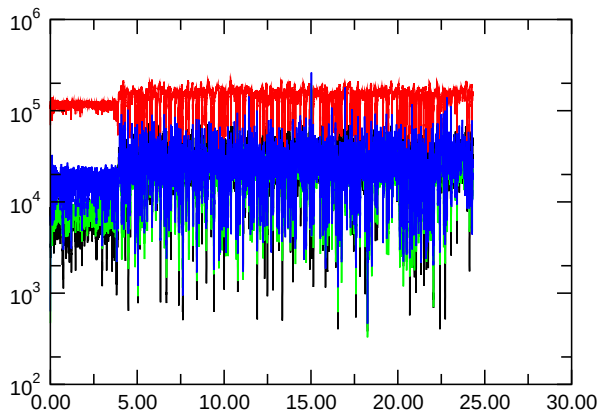
E_{kin,symm.}
