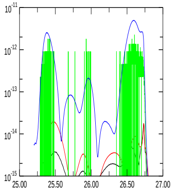
E_{\text{kin, asym}}
