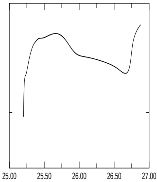
E_{\text{kin, asym}}
