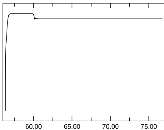
E_{\text{kin,asymm.}}
