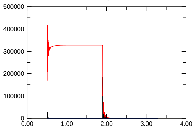
E_{\text{kin,symm.}}
