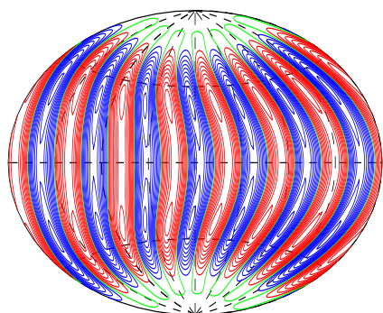
u_r (equat)
