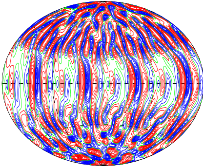
u_r (equat)
