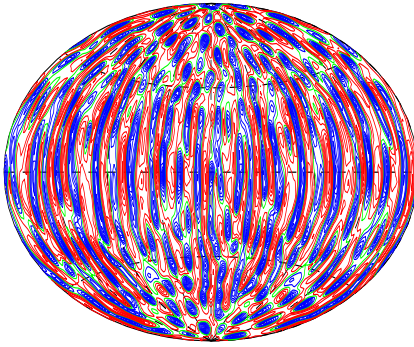
u_r at r = 0.5 (last snapshot)
