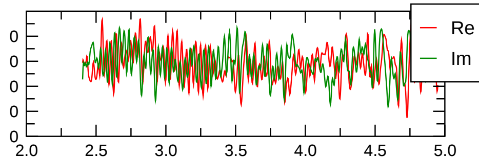
tor( m=0 ) magn.
