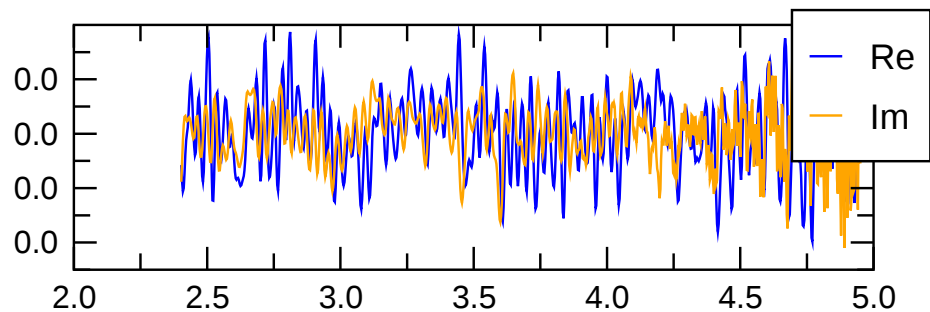
pol( m=1 ) magn.
