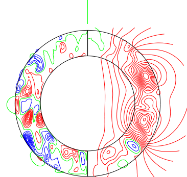
\bar{B}_\varphi & pol f-lines (mer)
