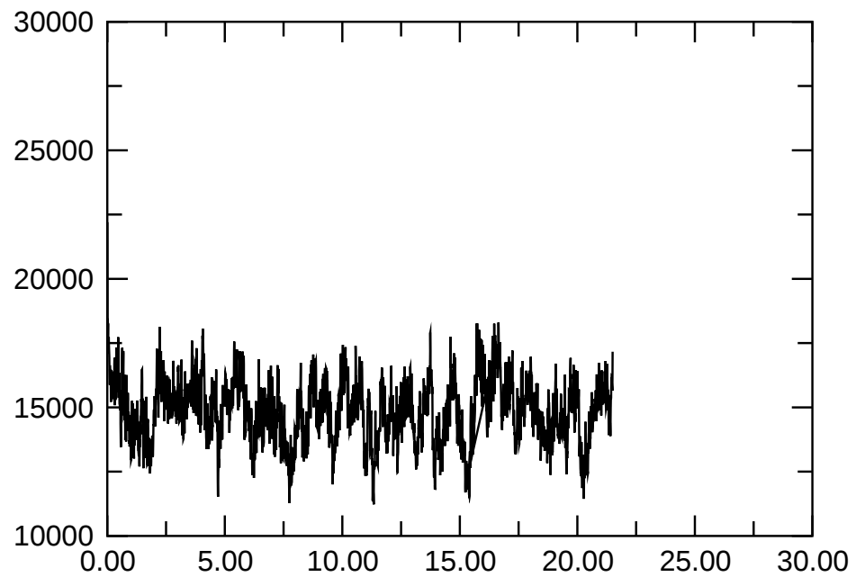
E_{\text{magn,quadr.}}
