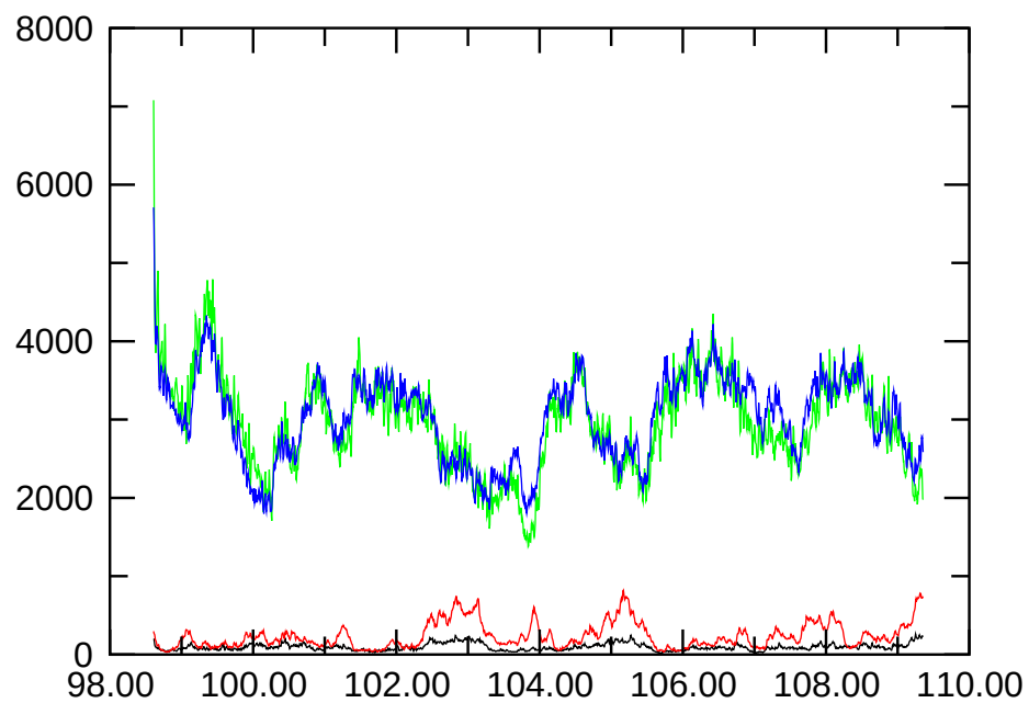
E_{\text{magn,quadr.}}
