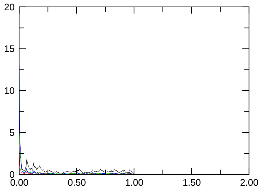
E_{\text{magn,quadr.}}
