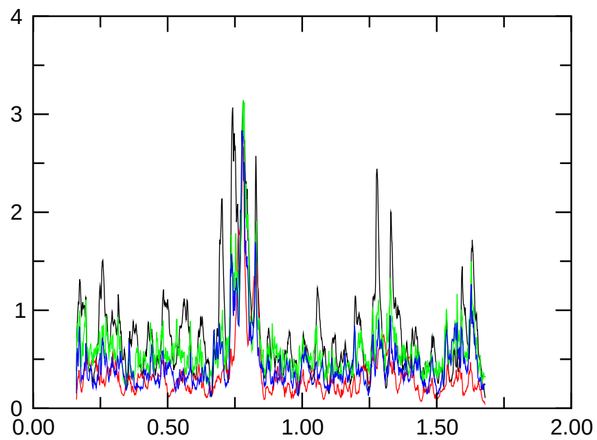
E_{\text{magn,quadr.}}
