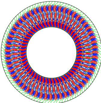
u_r (equat)
