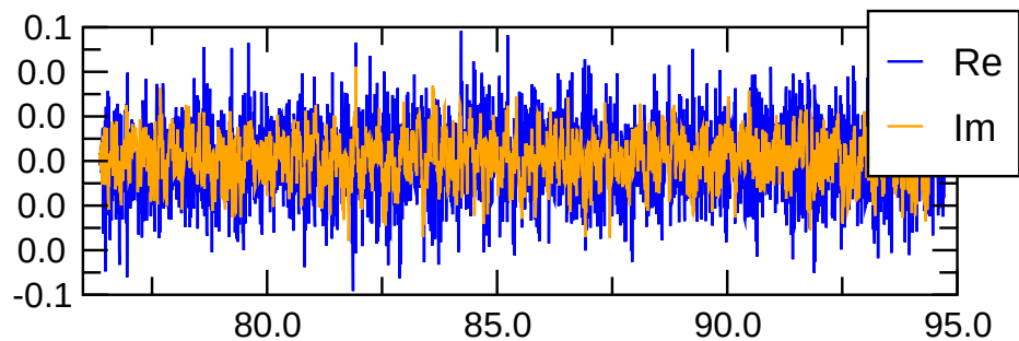
pol(m=1) magn.
