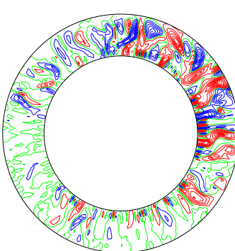
B_r (equat)
