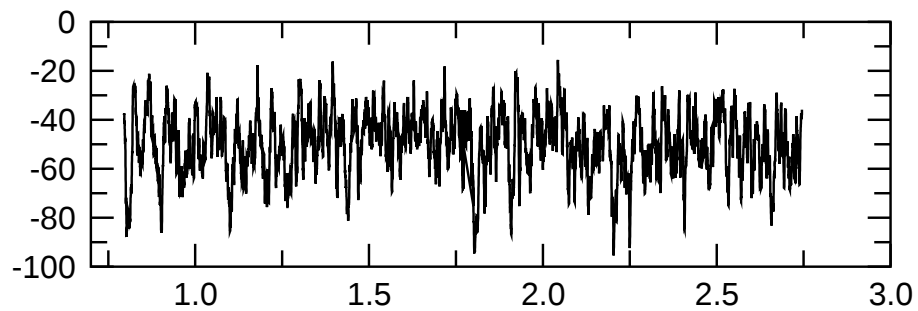
m=2 kin.
