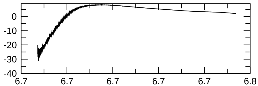
m=2 kin.
