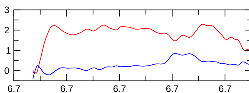
pol(m=0) magn.
