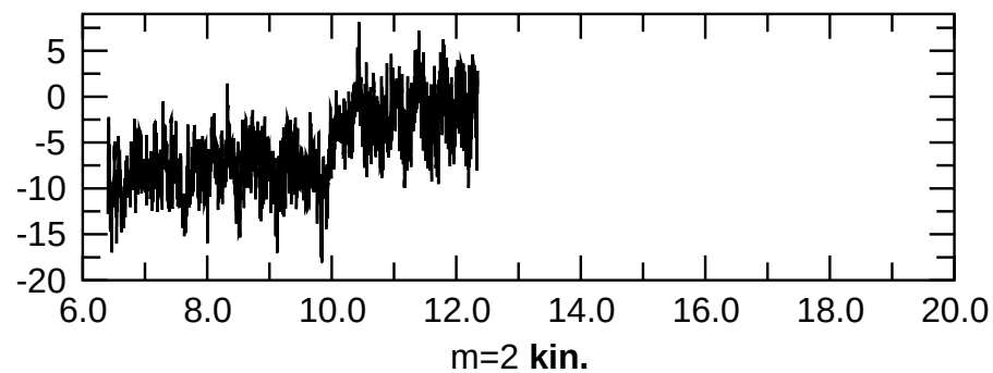
tor(l=1,m=0) kin.
