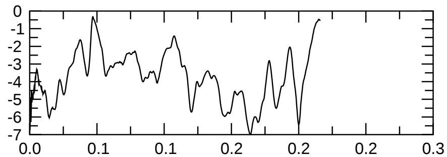
m=2 kin.
