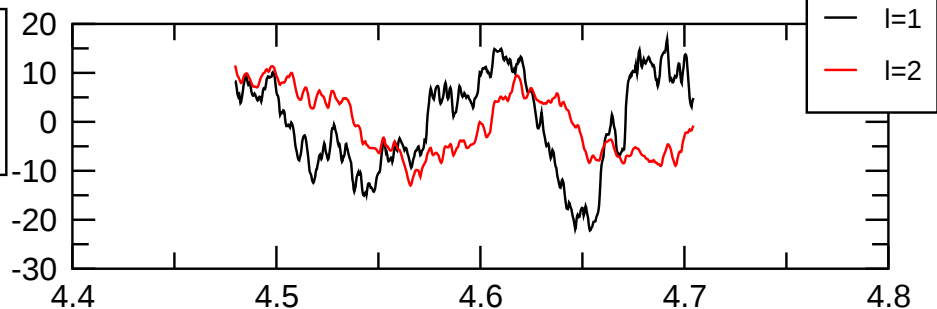
pol(m=2) magn.
