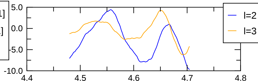
pol(m=0) magn.
