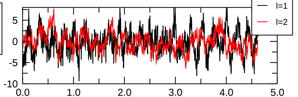
pol(m=2) magn.
