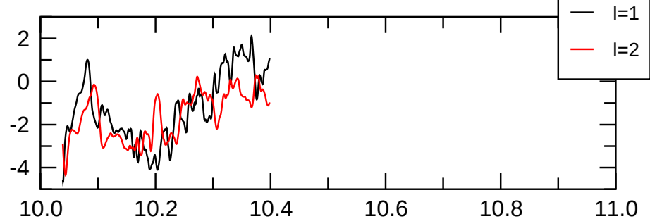
pol(m=2) magn.
