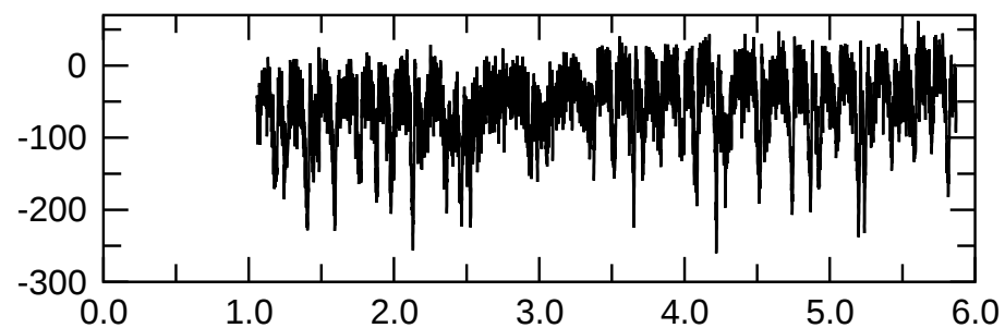
m=2 kin.
