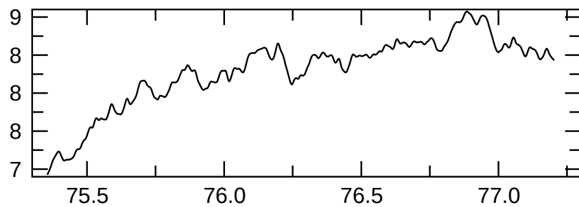
tor( l=1, m=0 ) kin.
