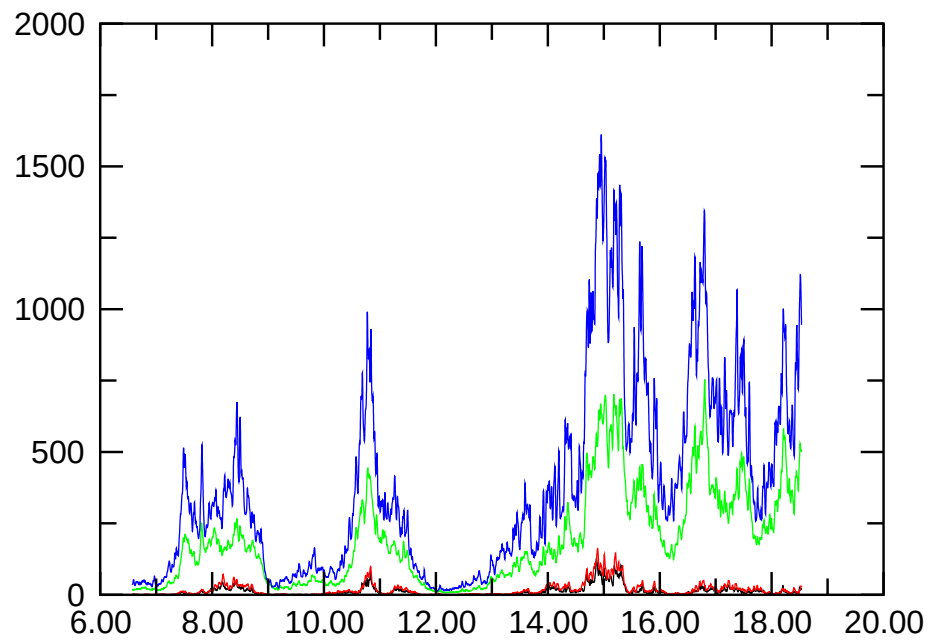
E_{\text{magn,quadr.}}
