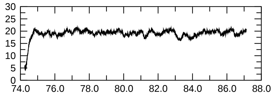
tor(l=1,m=0) kin.
