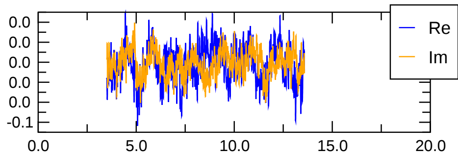
pol(m=1) magn.
