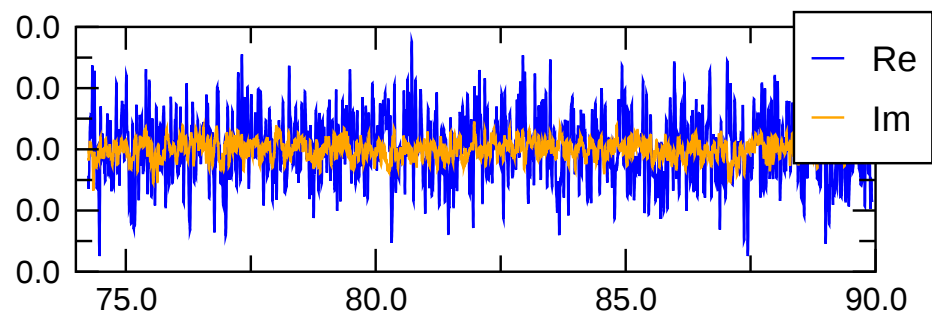
pol(m=1) magn.
