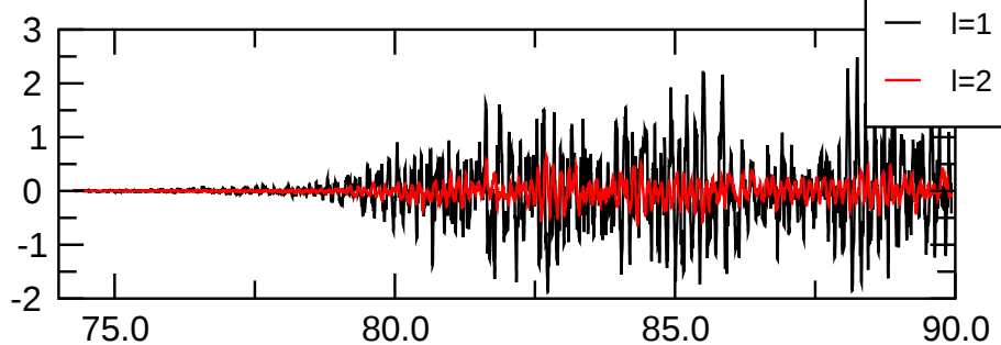
pol(m=2) magn.
