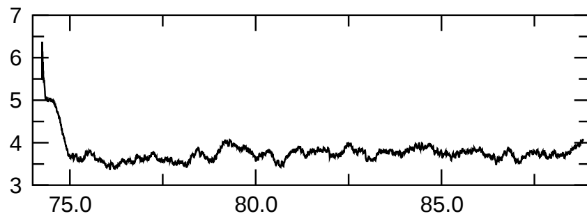
tor(l=1,m=0) kin.
