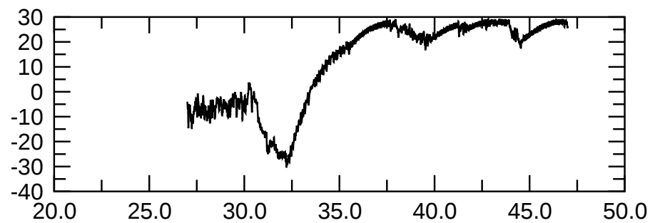
m=2 kin.
