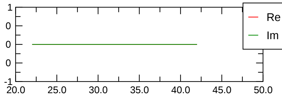
pol(l=1,m=1) kin.
