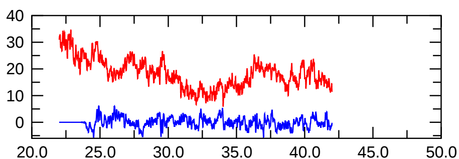
pol(m=0) magn.
