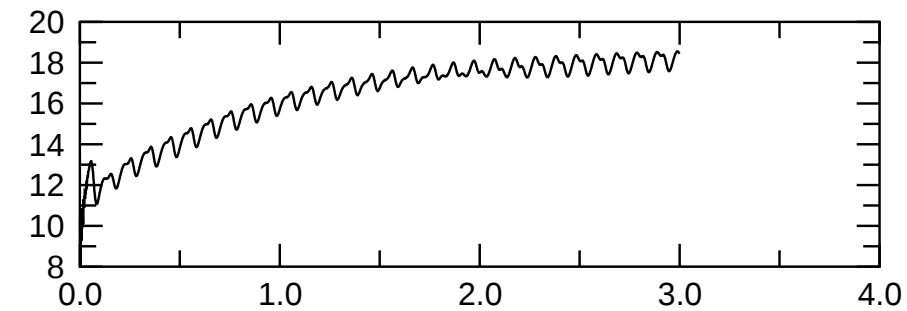
m=2 kin.
