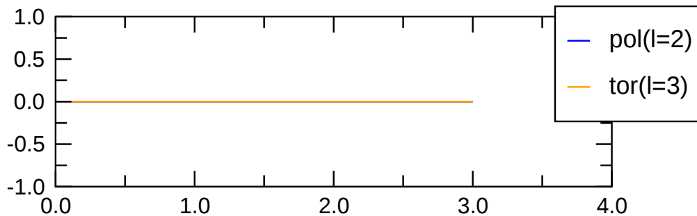
pol(m=1) magn.
