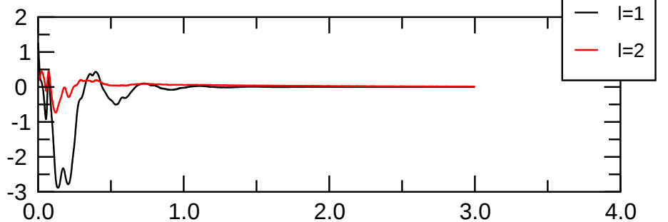
pol(m=2) magn.
