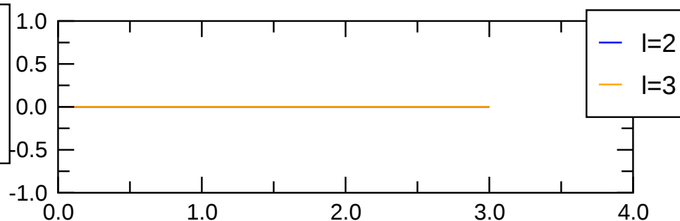
pol(m=0) magn.
